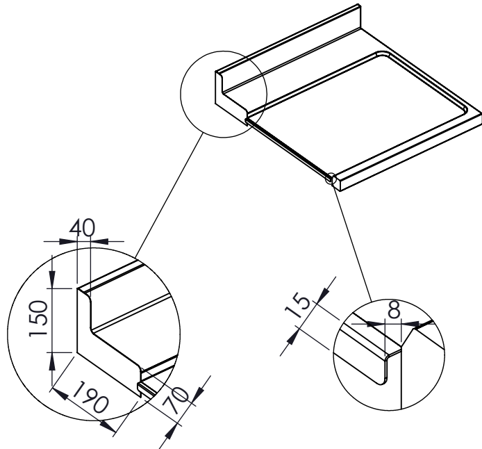
DETTAGLIO SCALA 1 : 2
